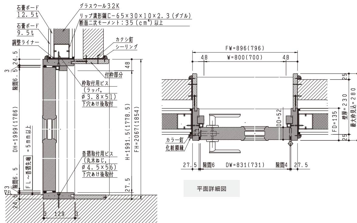
断面詳細図
