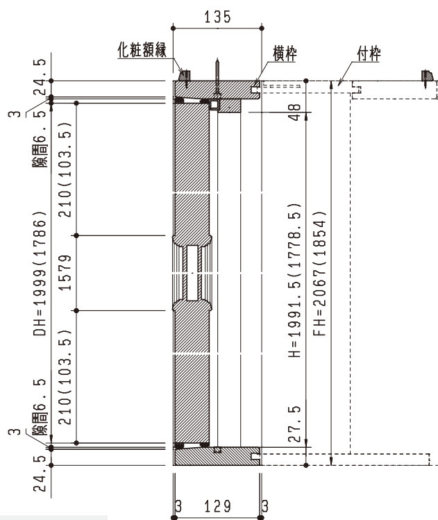
断面詳細図
