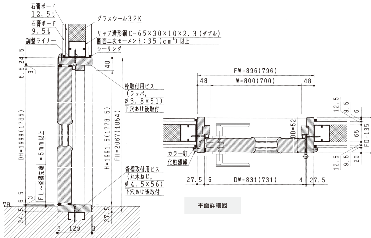
断面詳細図
