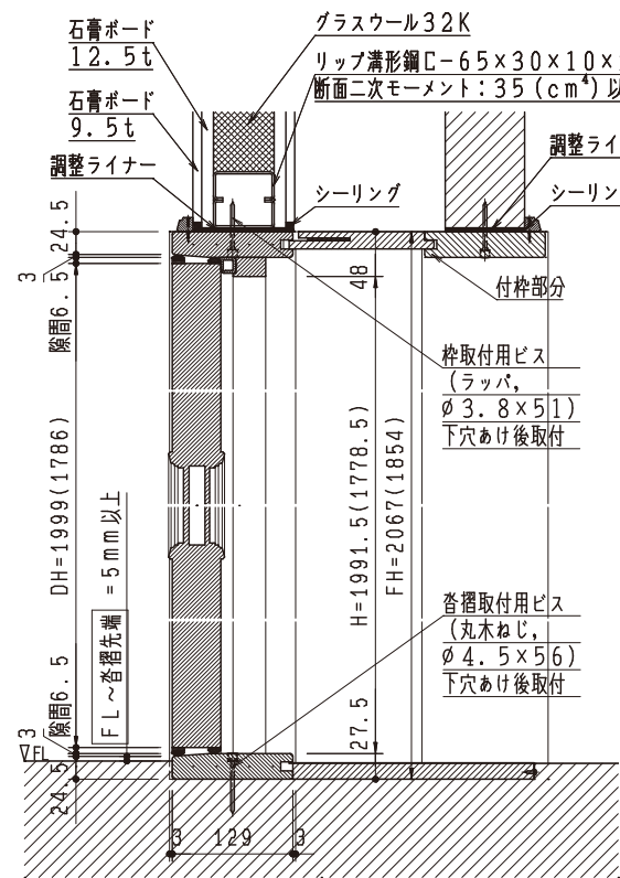
断面詳細図
