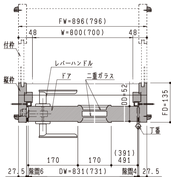
平面詳細図
