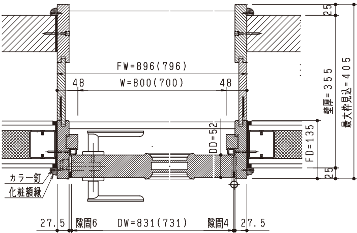
平面詳細図
