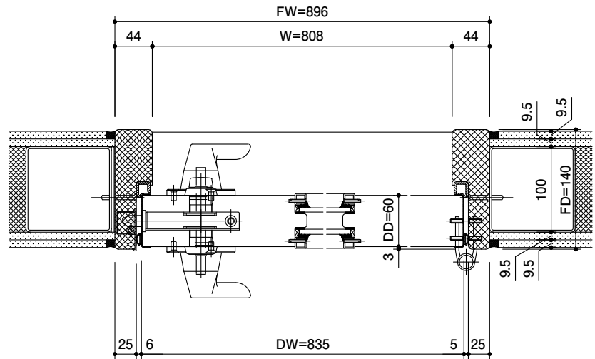
平面詳細図
