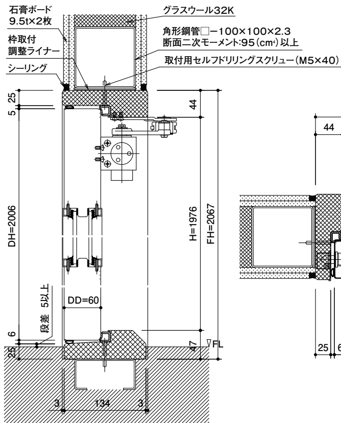
断面詳細図
